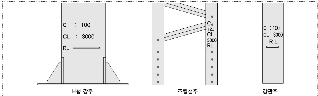
그림 1.3-1 일반철도 전철주 형식별 표기방법(예)
