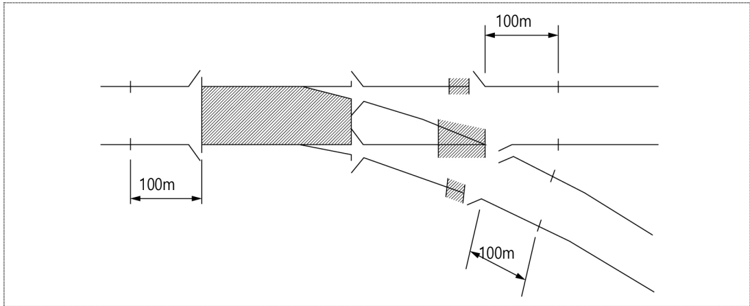
그림 2.3-2 절단한 레일 끝부분 틀어놓음
