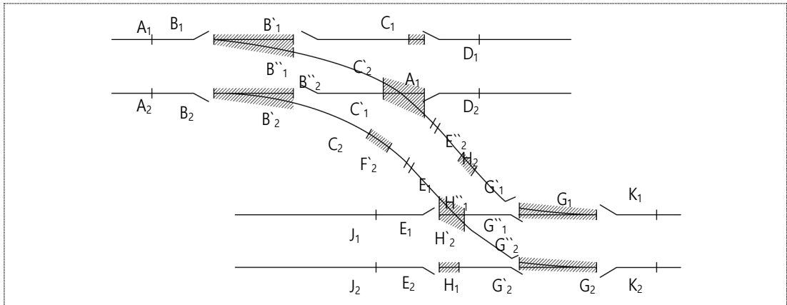
그림 2.3-4 건널선의 장대레일 재설정
