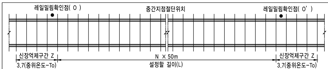
그림 1.3-1 레일인장기에 의한 장대레일 재설정
