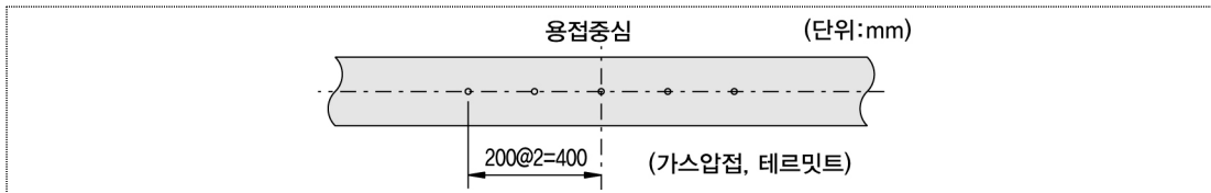
그림 1.3-5 경도 측정위치
