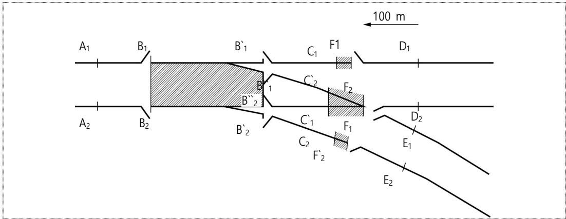
그림 2.3-3 편개 분기기의 장대레일 재설정
