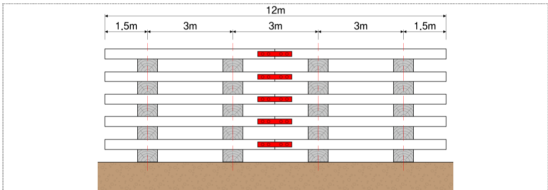
그림 3.1-1 접착절연레일 적치 및 목재받침대 배치 방법(12m 기준)
