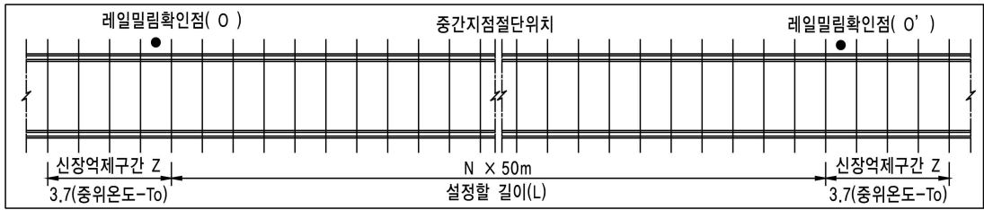
그림 2.3-1 레일인장기에 의한 장대레일 재설정
