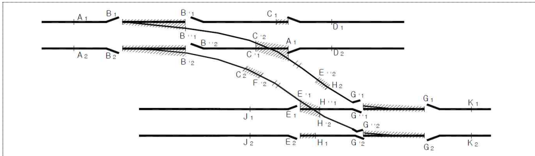
그림 3.3-4 건넌선의 장대레일 재설정
