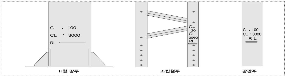
그림 3.3-1 일반철도 전철주 형식별 표기방법(예)
