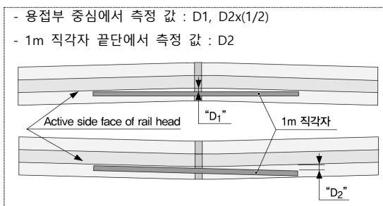
그림 1.3-2 줄맞춤 검사(방향, 줄틀림)
