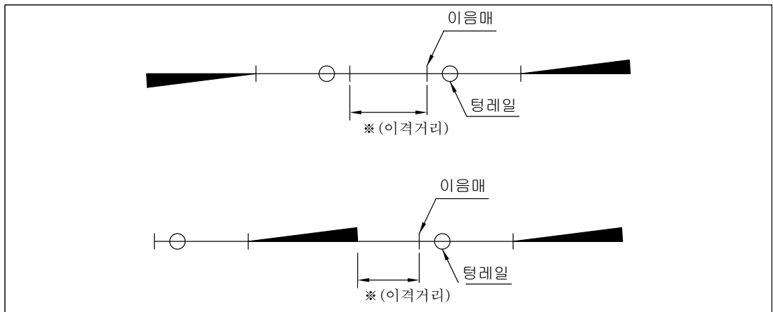
그림 3.3-1 분기기간 이격거리
