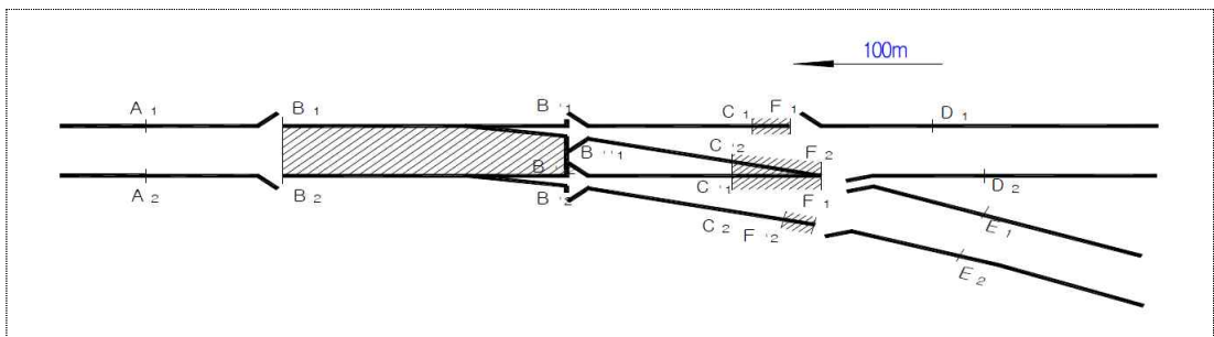
그림 3.3-3 편개 분기기의 장대레일 재설정
